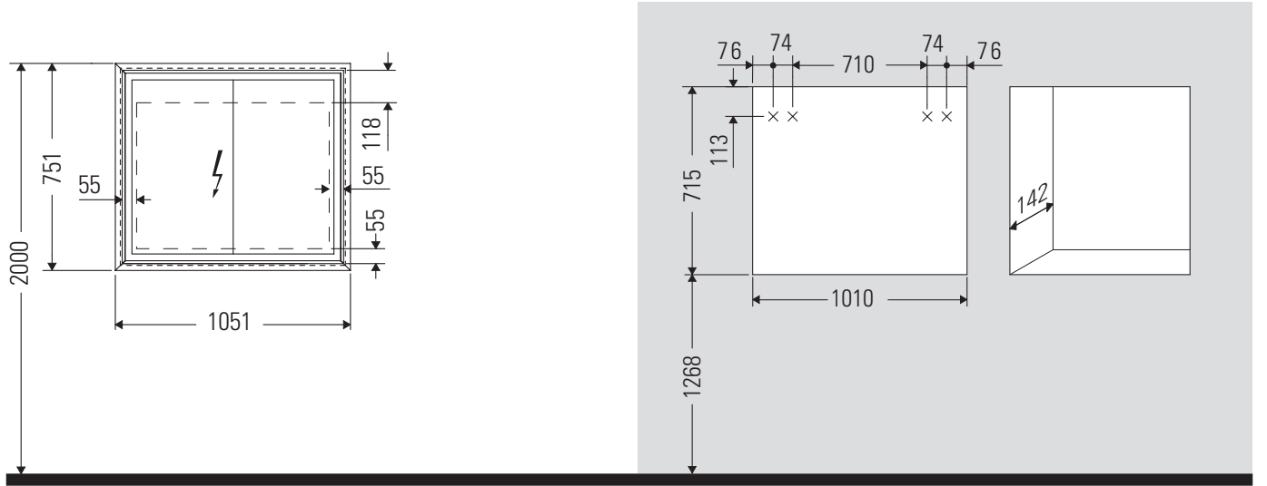
Ankastre dolaplar için açıklık ebatları
